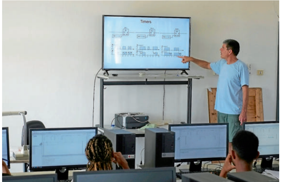
Reto Lüthin erklärt die vorhandenen Funktionen um die SPS Module zu programmieren Fotos: Jeremias Pellaton
